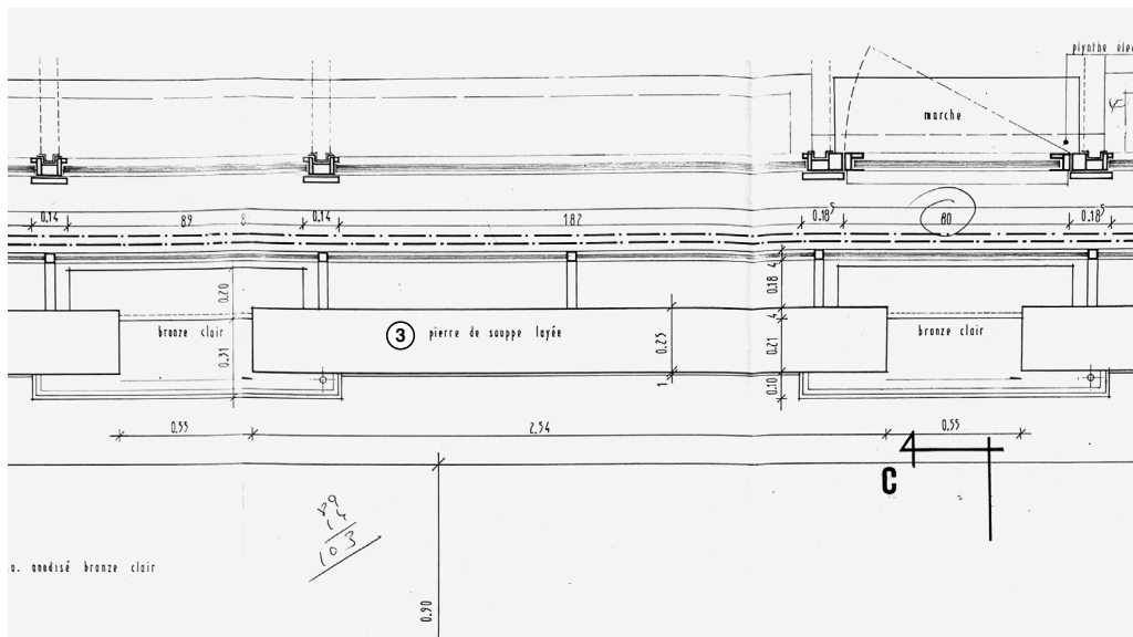
DÉTAIL Plan échelle 1/25
